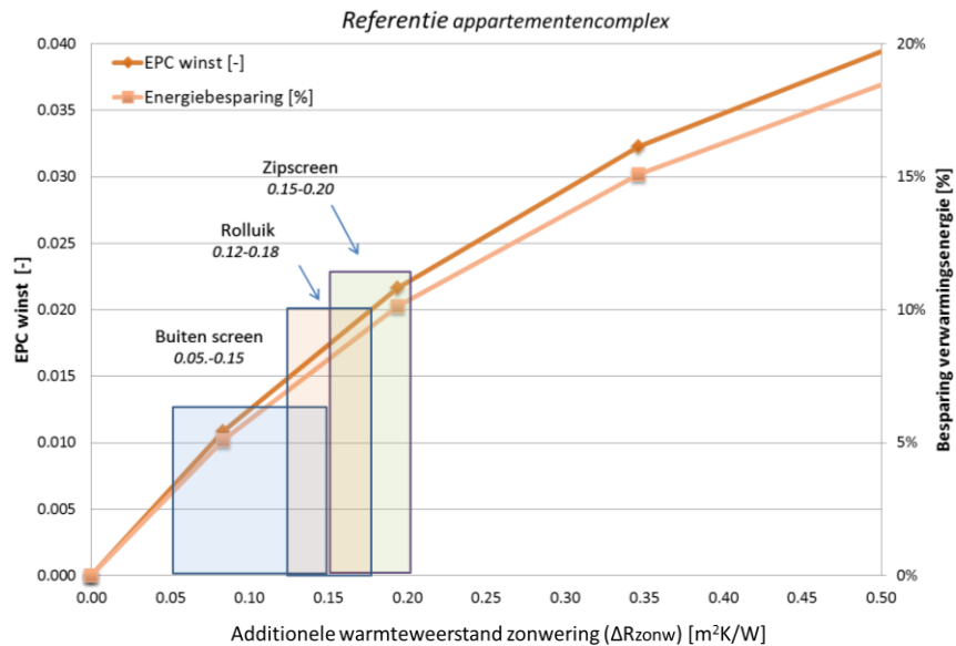
Figuur 14: Energiebesparing op verwarmingsenergie en potentiële EPC-winst door verschillende typen buitenzonwering voor het referentie appartement.
